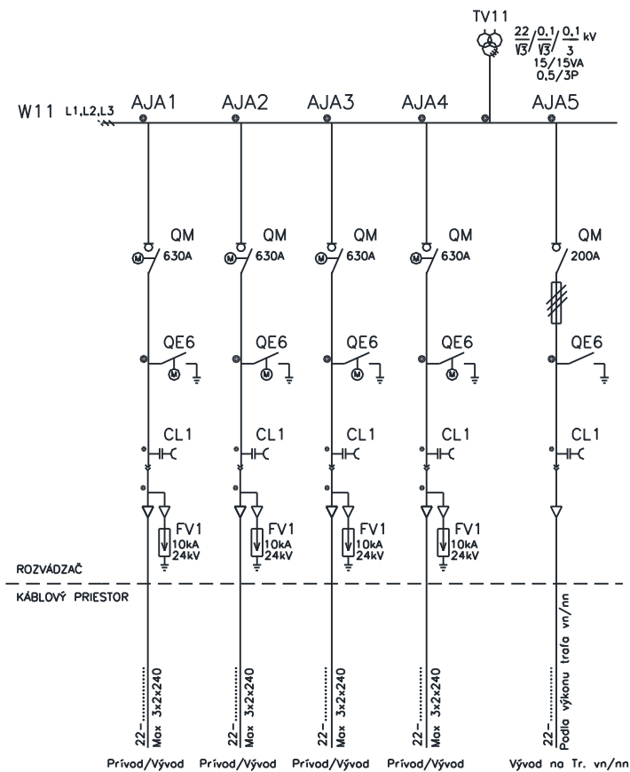
TS vn/nn Uzlová s Vnútným a diaľkovým ovládaním Jednopolová schéma 22 kV rozvádzača – Var.4
