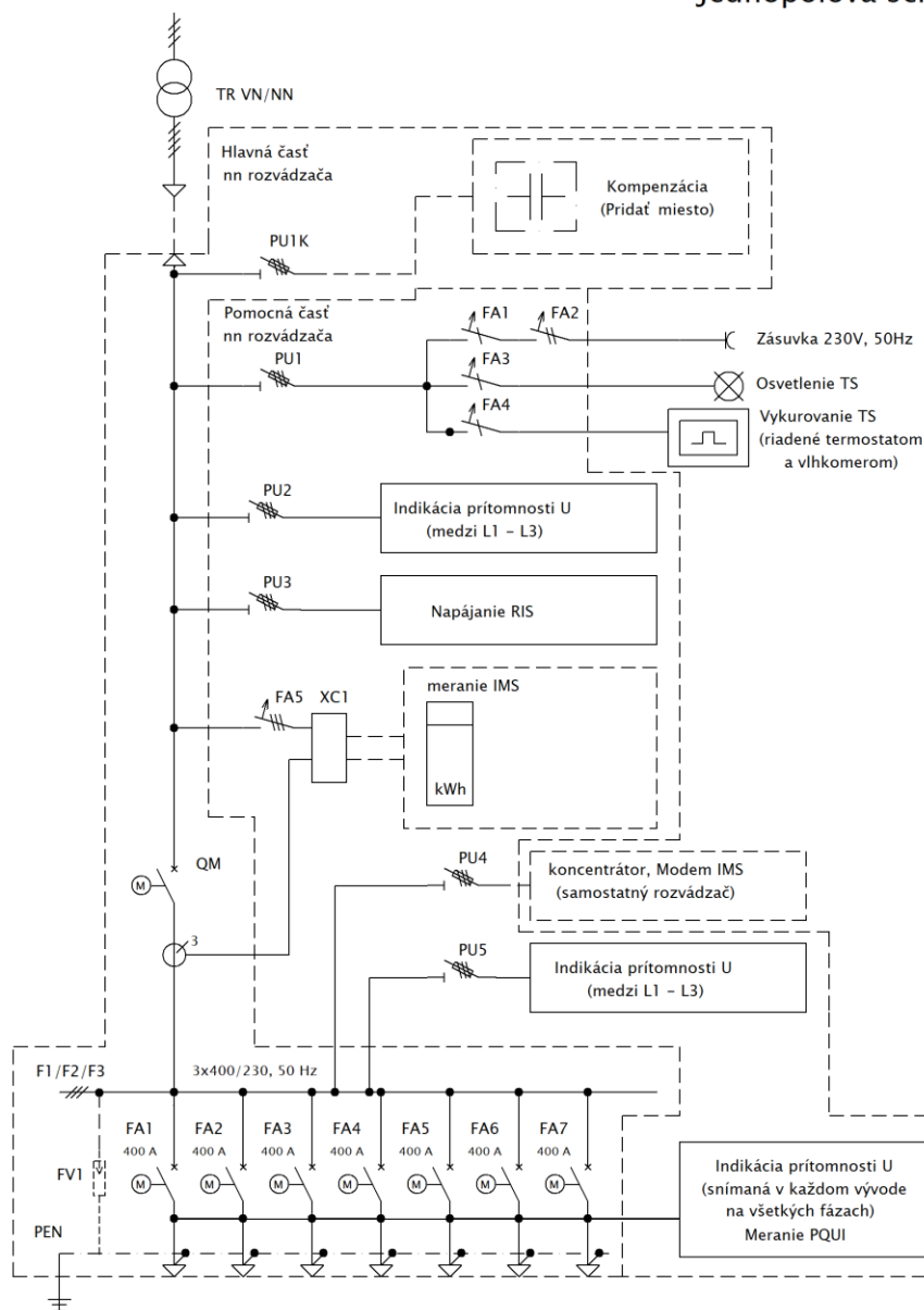
Jednopolová schéma NN rozvádzača var.1
