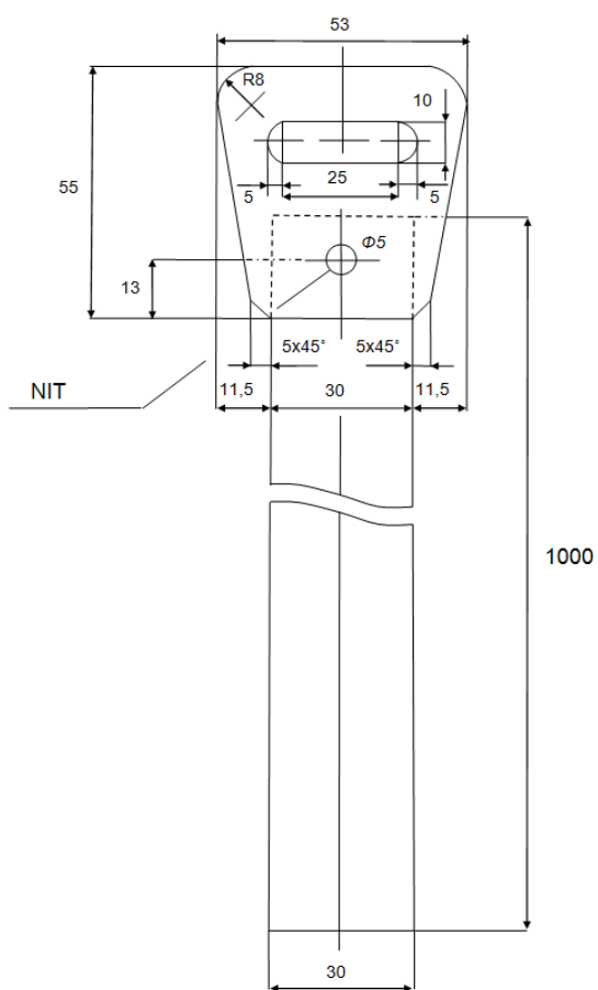
Obr. 3 Upínacia páska typu B
