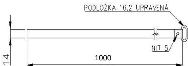
Obr. 1 Upínacia páska typu A
