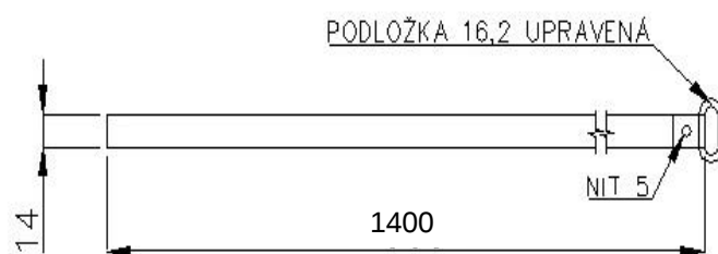
Obr.2 Upínacia páska typu C
